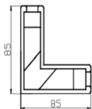
Squadretta di allineamento anta portoncino astro 6
