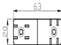
Squadretta di aggancio per zoccolo
