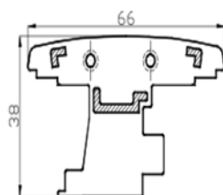
Terminale per profilo 16003
