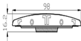
Terminale per profilo 19103
