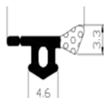
Guarnizione sormonto anta
