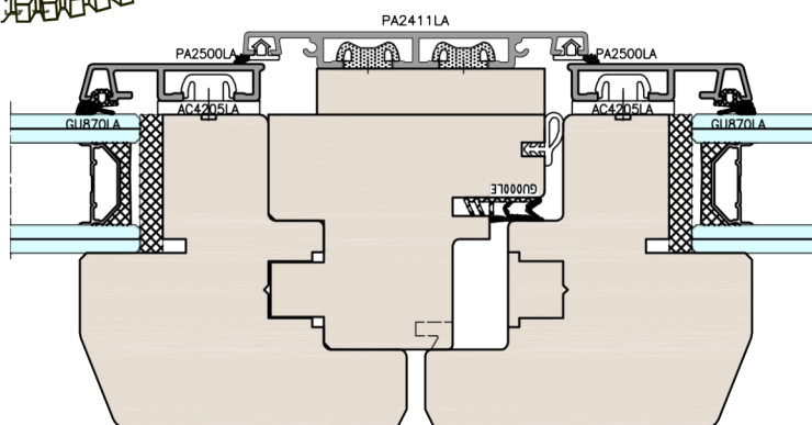
Snodo centrale ante asimmetriche
