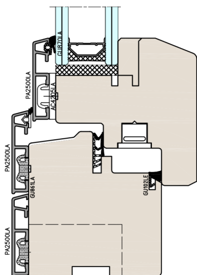
Snodo inferiore
