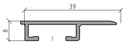
PA2501LA - PROFILO ANTA VETRO
