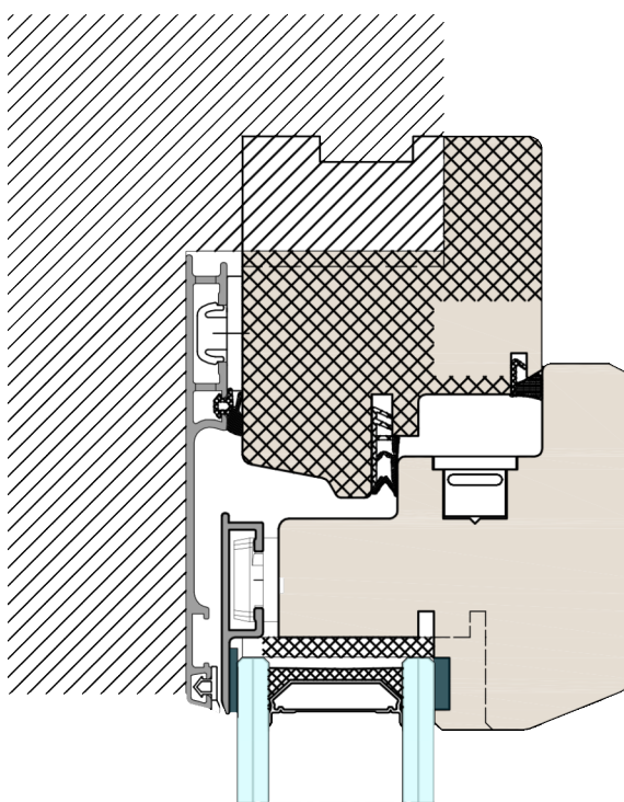
SOLUZIONE LEGNO VETRO INCASSO TOTALE ANTA FILO MURO
