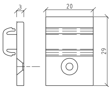
AC4208LA - CLIP BLOCCAGGIO ANTA-VETRO
