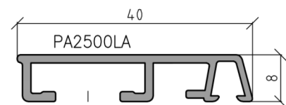
PA2500LA - PROFILO ZOCCOLO/ANTA
