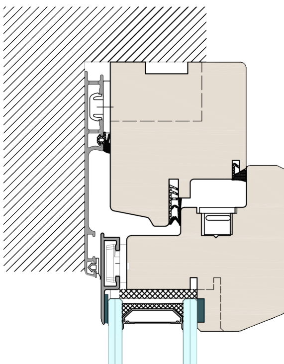
SOLUZIONE LEGNO VETRO TELAIO INCASSATO
