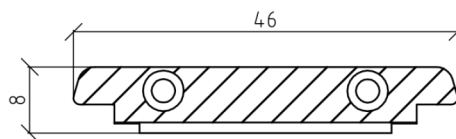
AC4213LA — TERMINALE PER PROFILO PA2424LA
