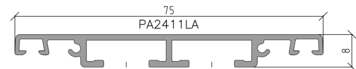
PA2411LA - PROFILO MONTANTINO
