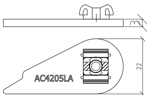
AC4205LA - CLIP BLOCCAGGIO SCATTO
