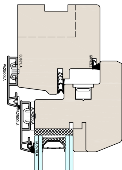
Snodo superiore
