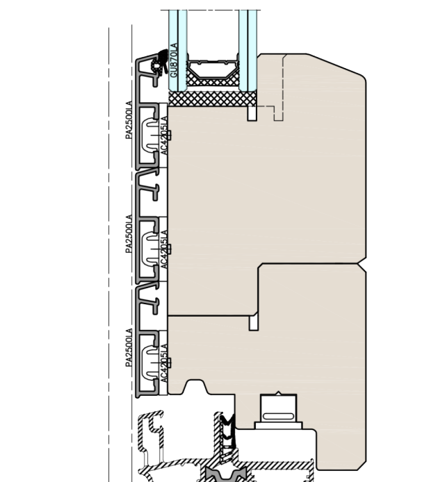
Snodo inferiore portabalcone
