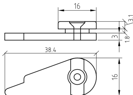
AC4520LA - CLIP BLOCCAGGIO MANUALE
