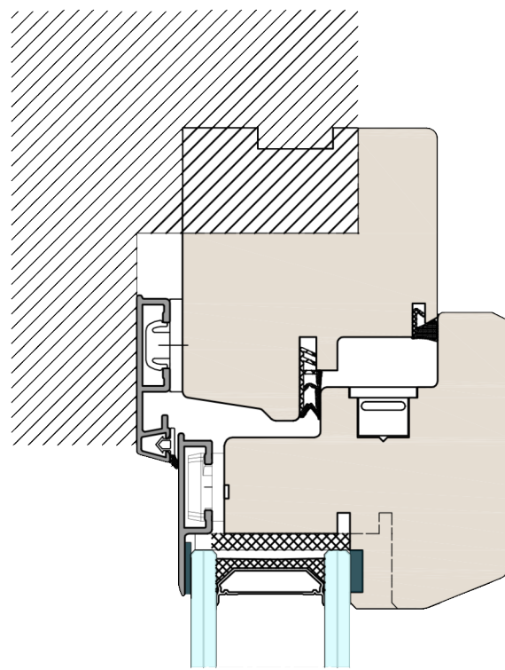
TELAIO A SBALZO ANTA MINIMALISTA
