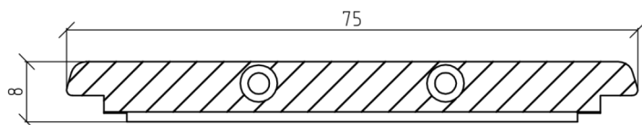
AC4212LA — TERMINALE PER PROFILO PA2411LA
