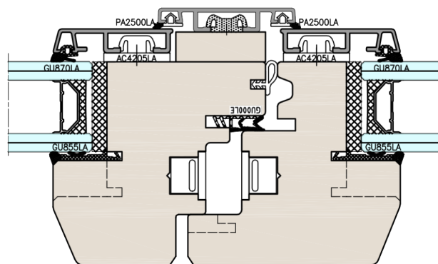
Snodo centrale ante simmetriche
