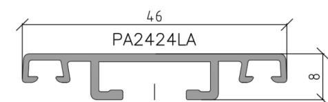
PA2424LA - PROFILO MONTANTINO
