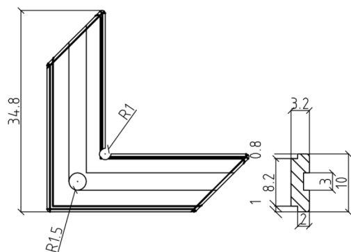
AC4215LA - SQUADRETTA ALLINEAMENTO
